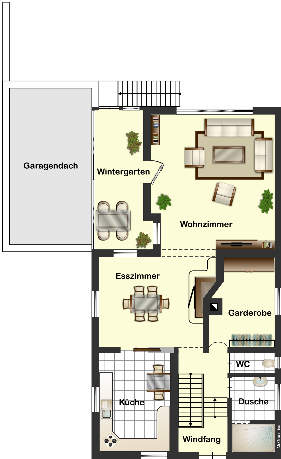
Erdgeschoss
