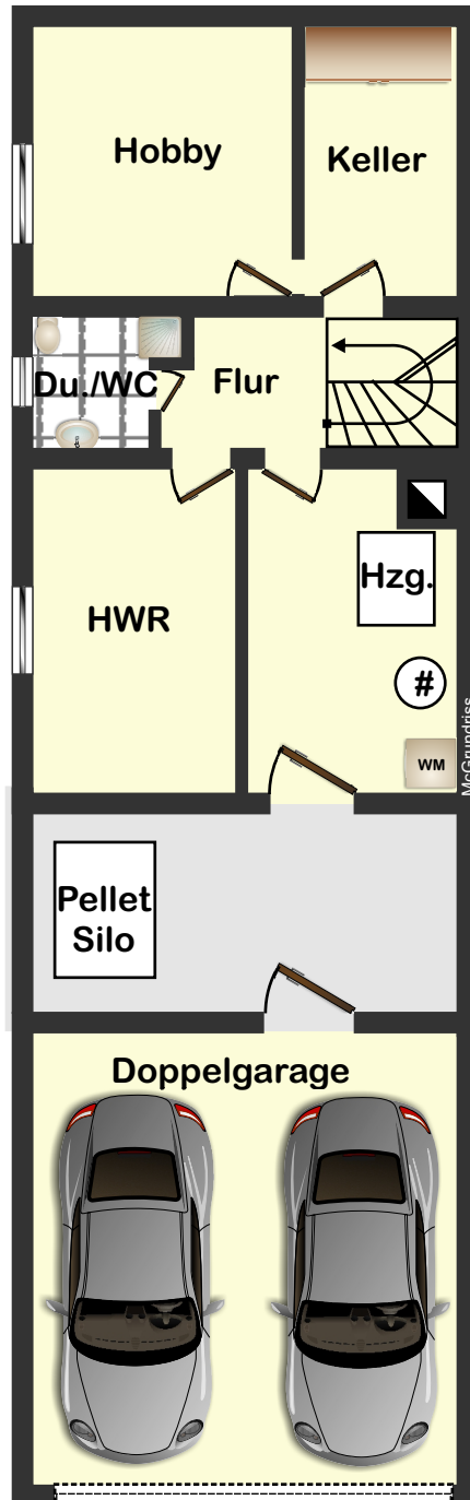
Untergeschoss
